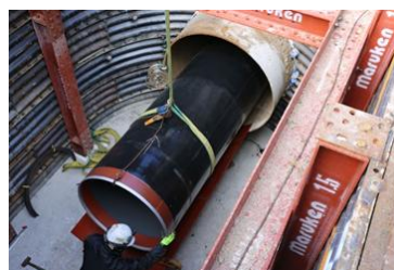
耐震化（パイプインパイプ工法）
