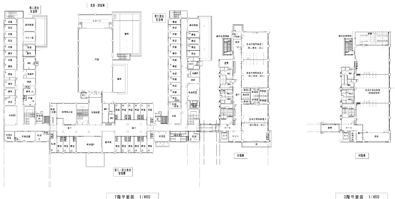
2階平面図 1/400
