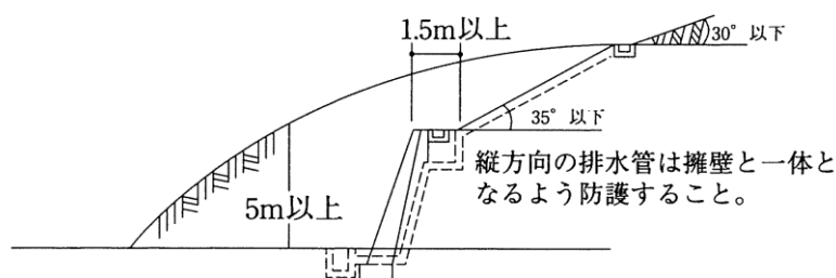
図 4-3 のり肩排水溝の例
