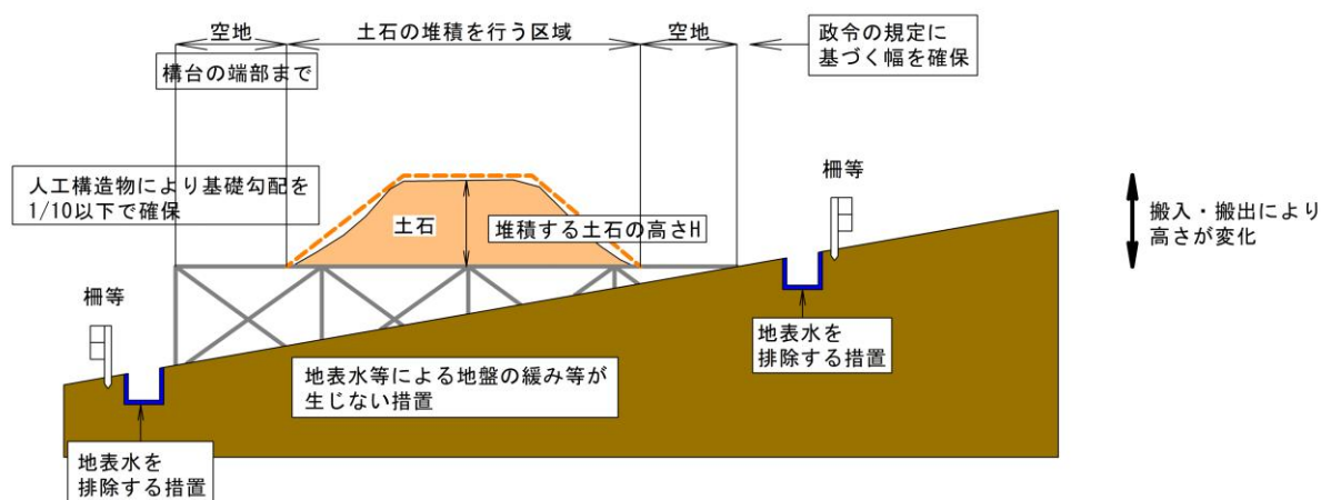
図 6-3 堆積した土石の崩壊やそれに伴う流出を防止する措置（地盤勾配が 10 分の 1 を超える場合） 参考：盛土等防災マニュアルの改正概要と考え方(国土交通省、令和 5 年 5 月)、一部加工
