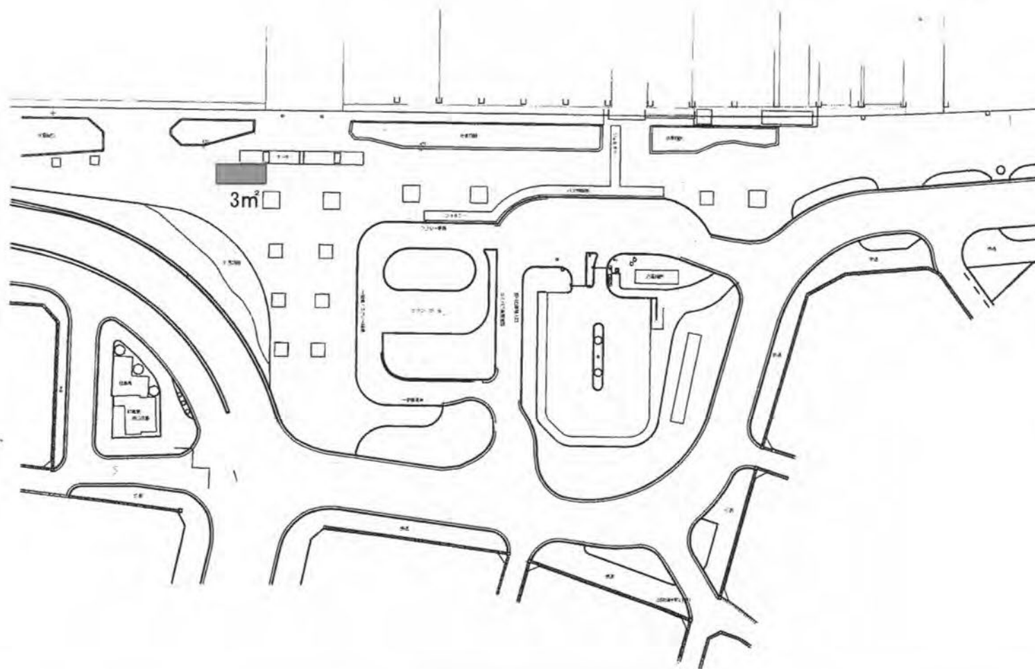
岐阜駅南口駅前広場平面図 S=1/500
