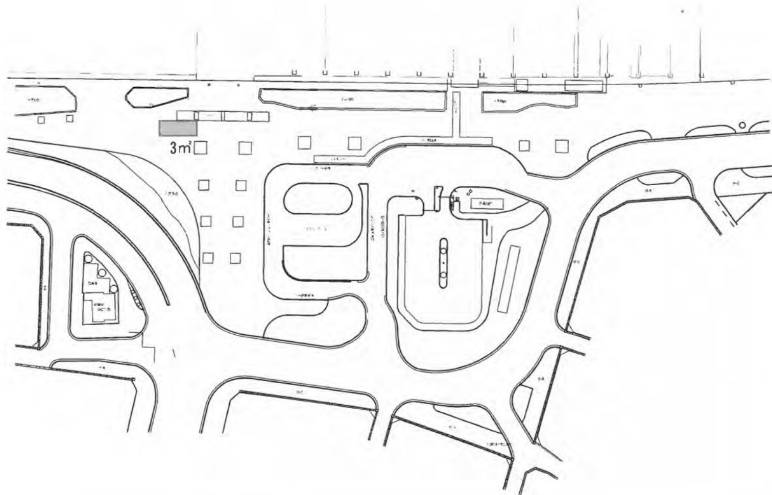
岐阜駅南口駅前広場平面図 5:1/500
