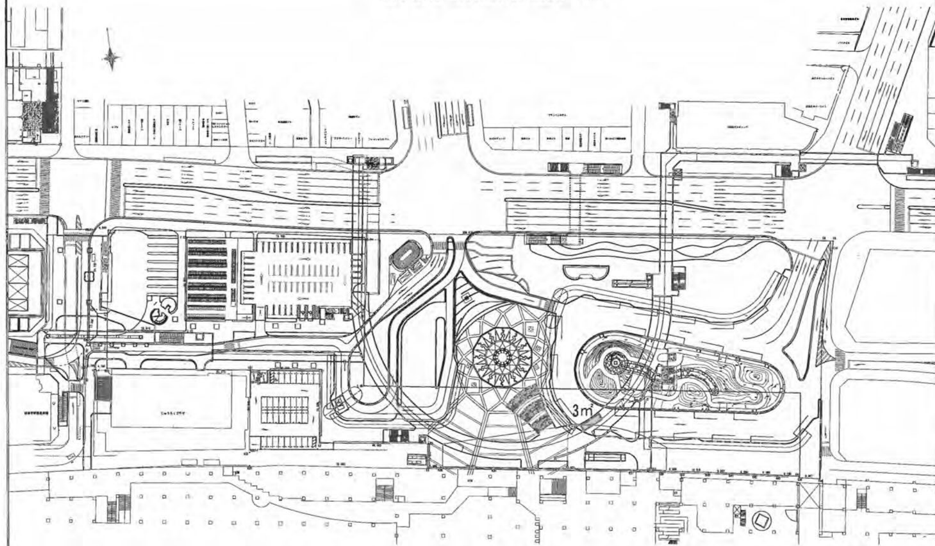
岐阜駅北口駅前広場平面図 S=1/500
