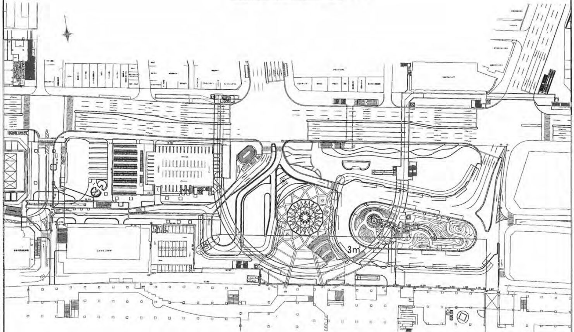
岐阜駅北口駅前広場平面図 S=1/500
