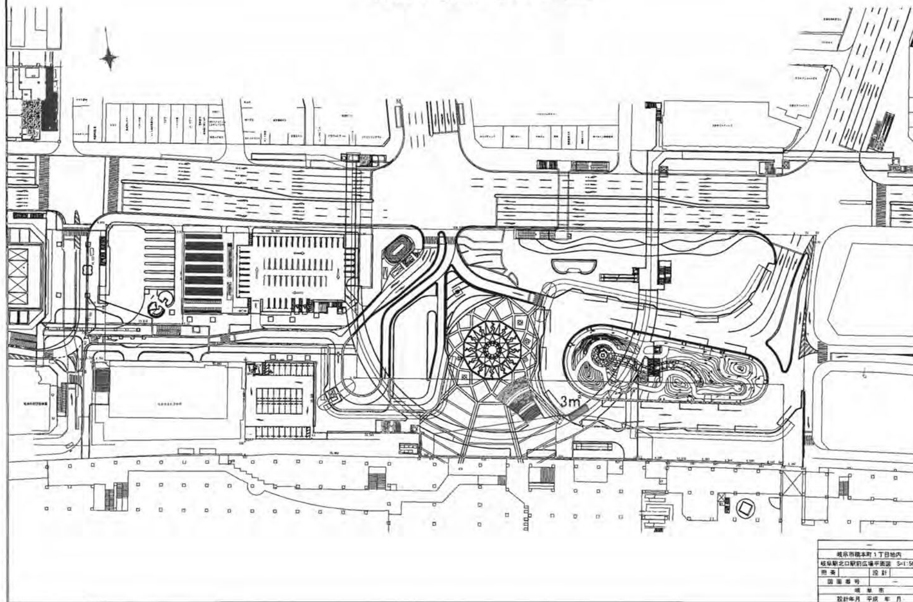
岐阜駅北口駅前広場平面図 S-1/500
