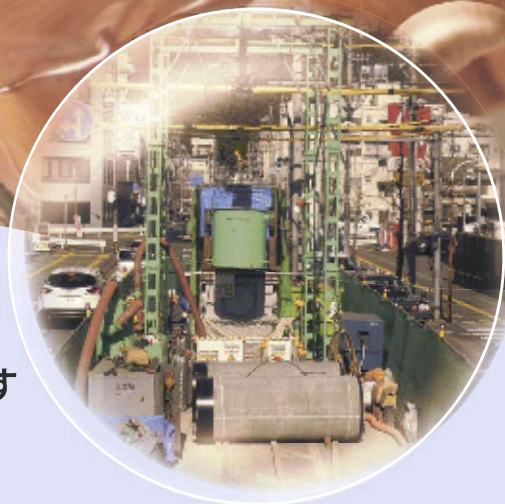
下水道幹線の耐震化工事
