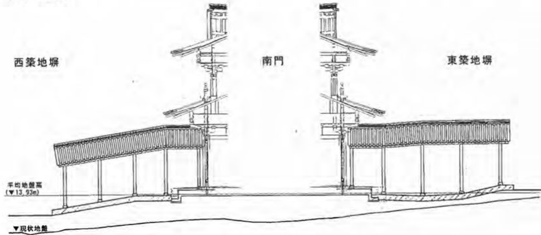
1 南立面
