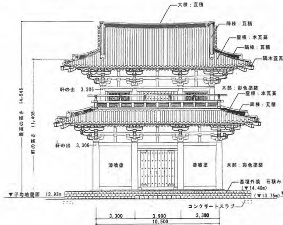
1 南立面図
