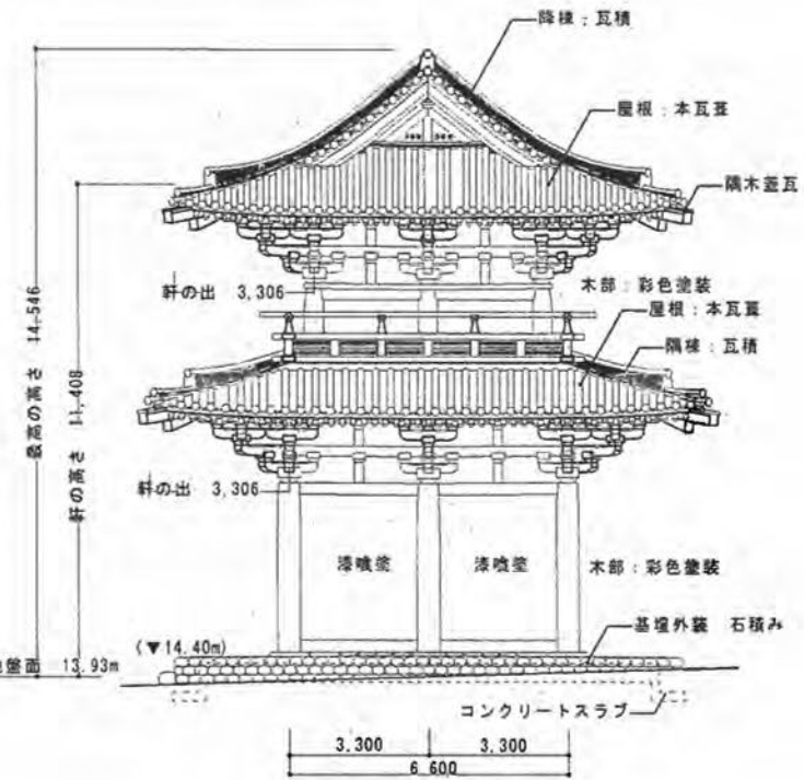
2 東立面図
