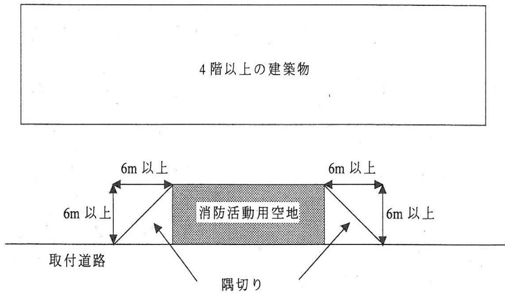
別図2 消防活動用空地と建築物の距離
