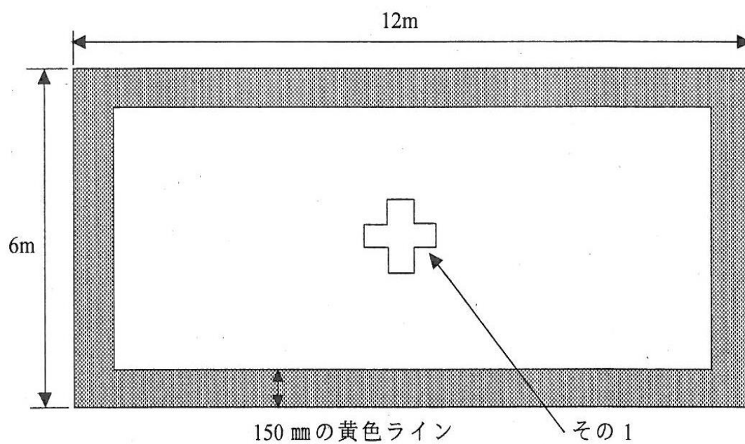
別図 3-1 消防活動用空地の規制表示
