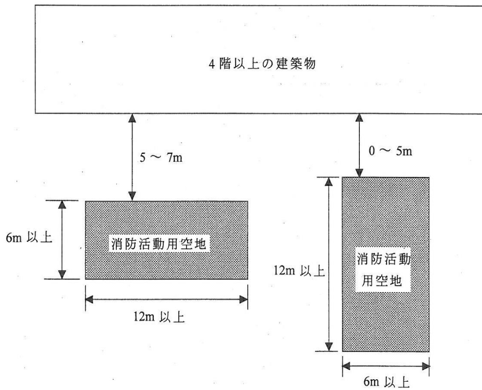
別図2 消防活動用空地と建築物の距離
