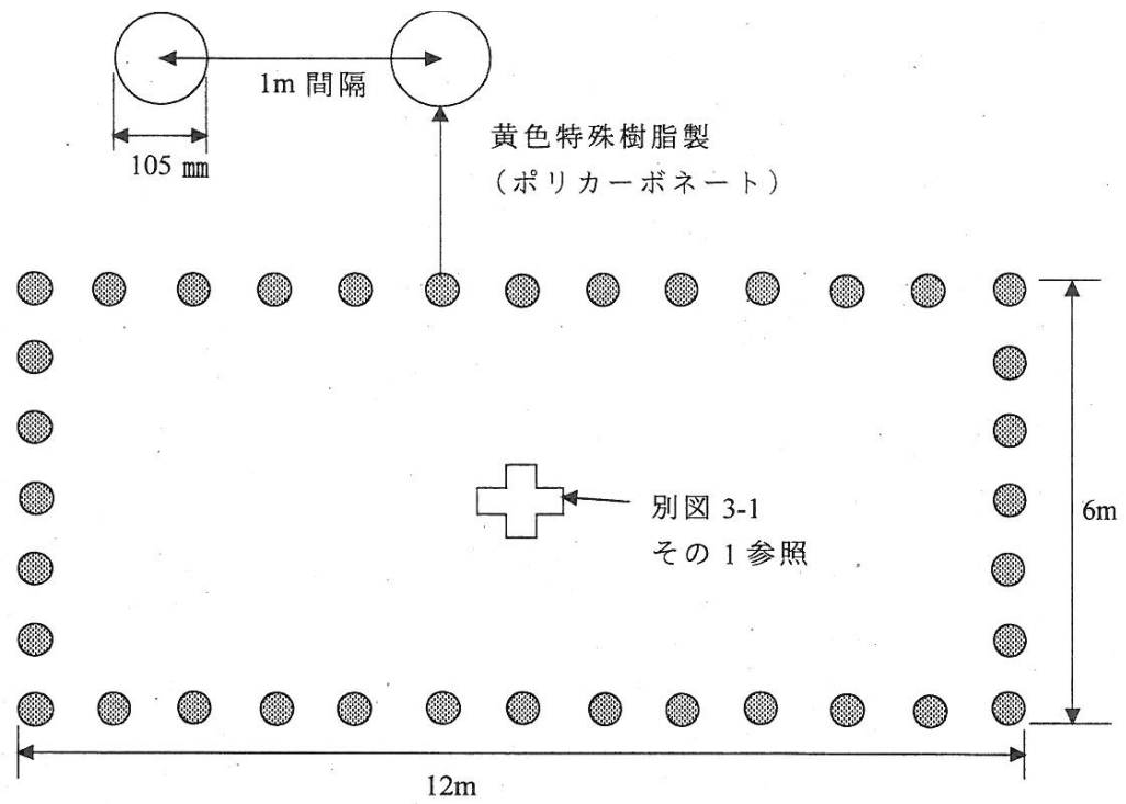
別図 3-2 消防活動空地の規制標示
