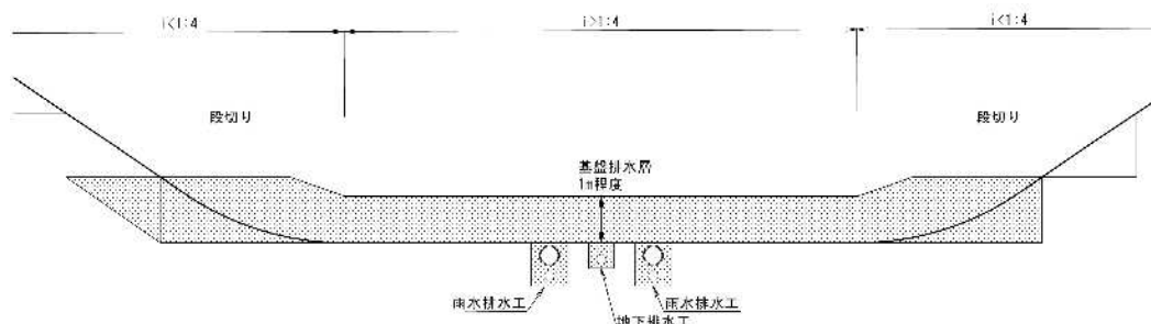
図 1-8 基盤排水層の設置例
