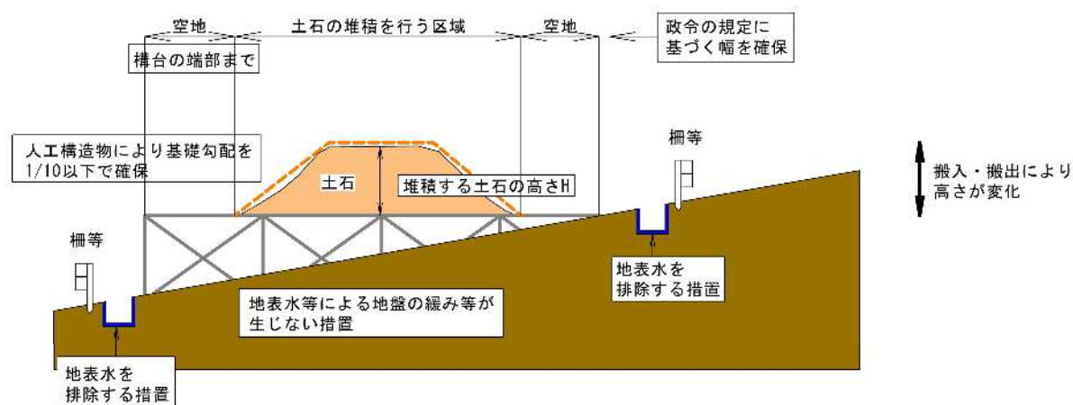
図 6-3 堆積した土石の崩壊やそれに伴う流出を防止する措置（地盤勾配が 10 分の 1 を超える場合）
