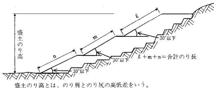
図 1-2 盛土のり高
