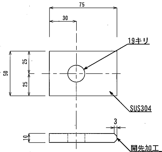
図1 ボイラ2パス用サポートラグ
