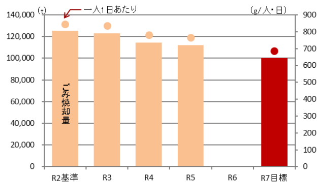
図-1 ごみ焼却量の推移
