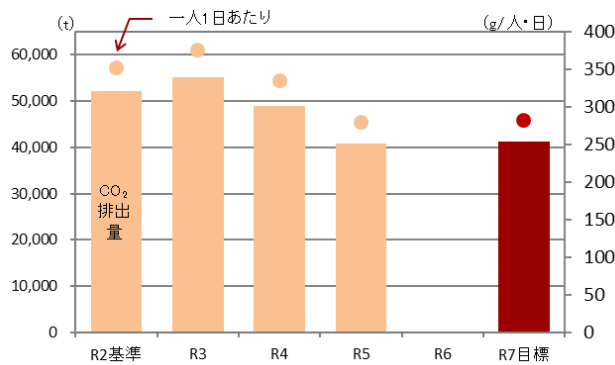
図-2 ごみ焼却による CO 2 排出量の推移
