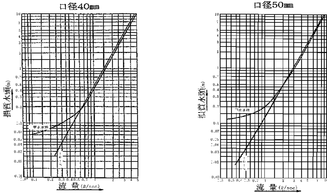
図30-5 水栓類、メーター類の損失水頭図表 ( \phi 40 、 50 mm)
