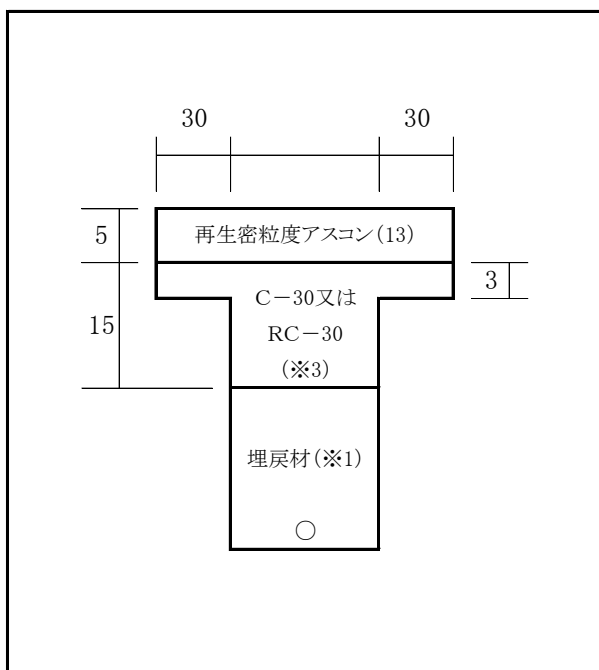
①加熱混合式舗装(L交通(簡易))
