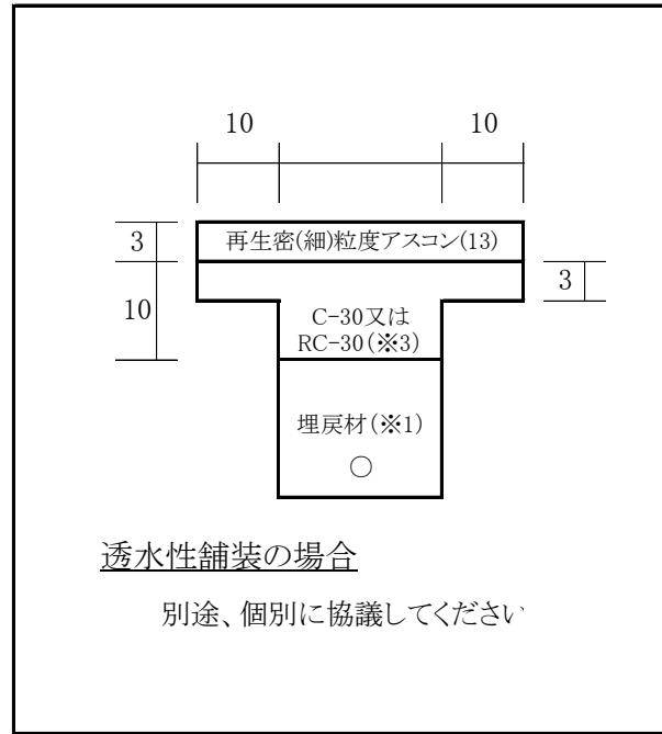
⑥加熱混合式舗装(歩道)
