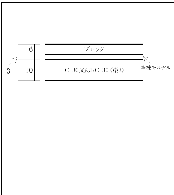
⑦コンクリートブロック舗装(歩道)
