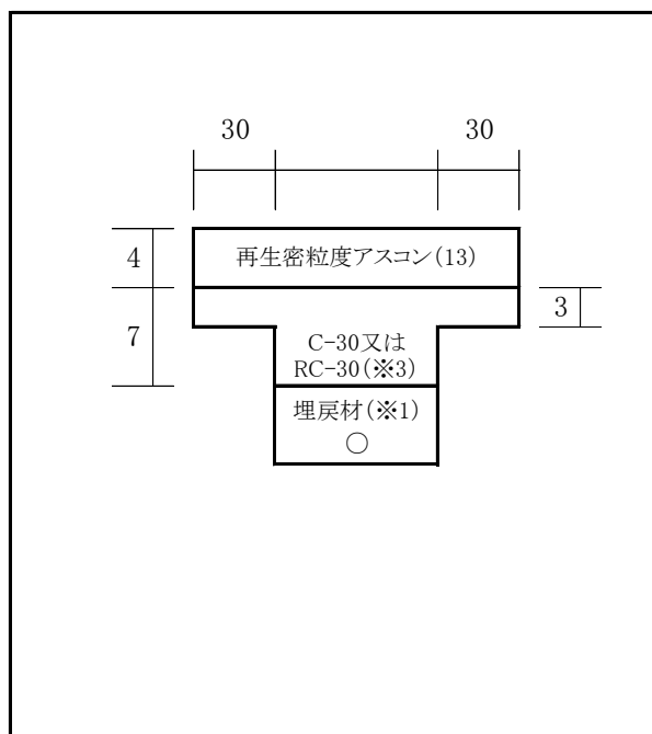
②浸透式マカダム舗装(現況)
