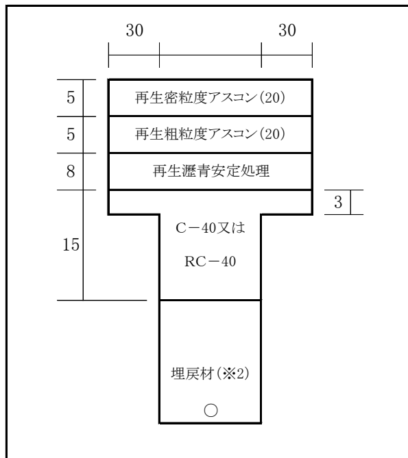
④加熱混合式舗装(C交通)
