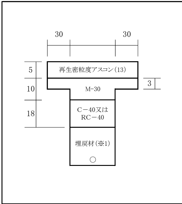
⑤加熱混合式舗装(L・A交通)
