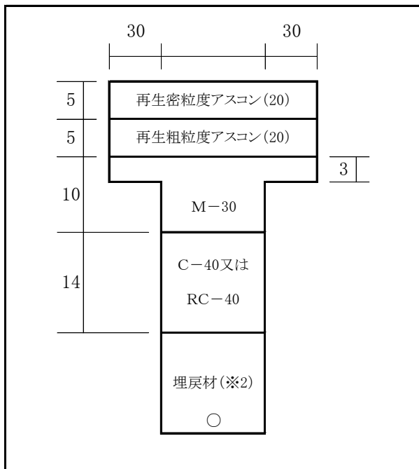
③加熱混合式舗装(B交通)
