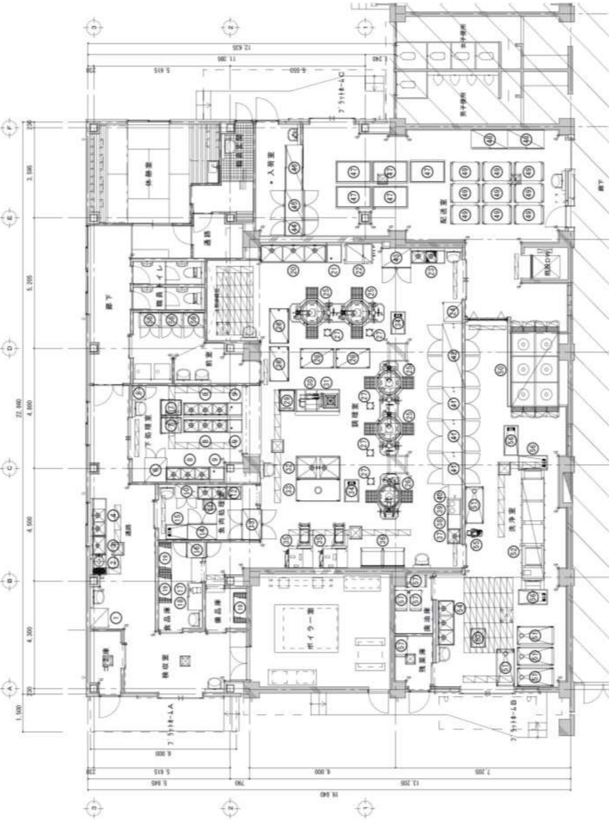
(参考)長良中学校給食共同調理場平面図
