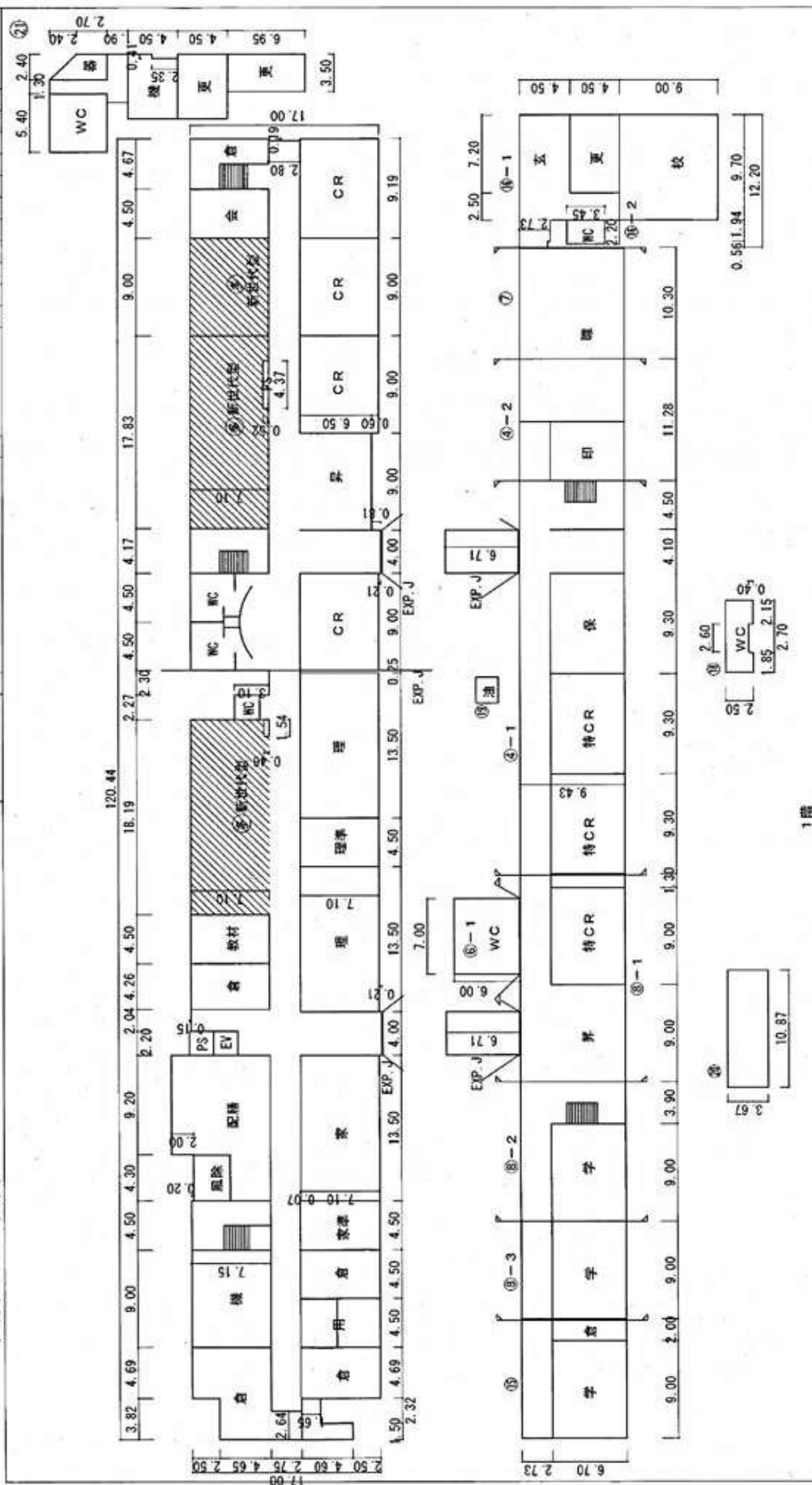
平面图 英尺 1/500 长良西小学校 西原町 21 201 0044 昭和33年
