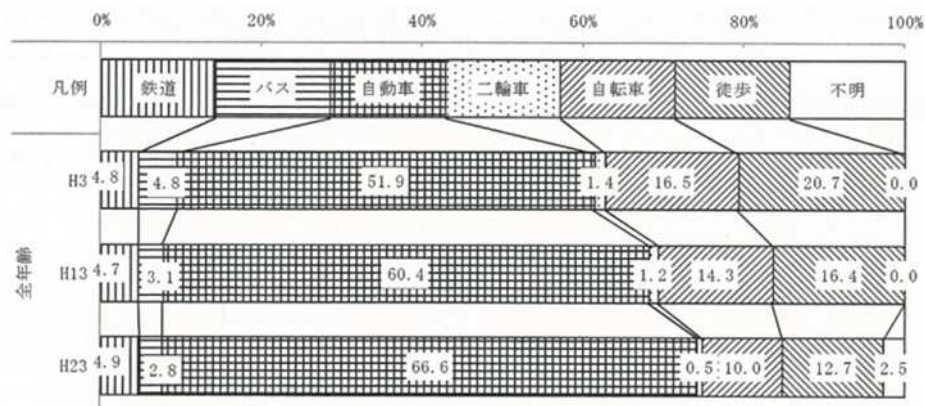
図 交通手段の比率
