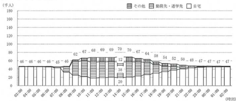
図 主要ゾーンの時刻別滞留人口（平日）
