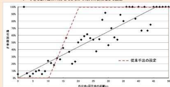
図 東日本大震災発生当日における外出距離別の帰宅困難率 (代表交通手段が鉄道の場合を抽出して分析)
