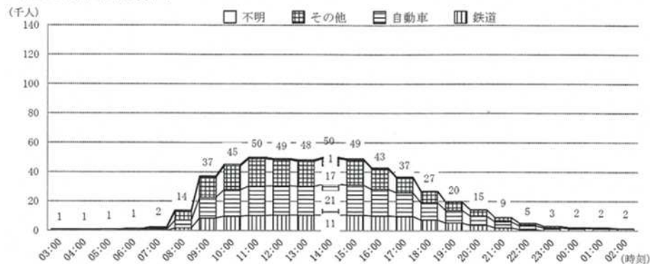
図 主要ゾーンの時刻別自宅発交通手段別滞留人口（平日）
