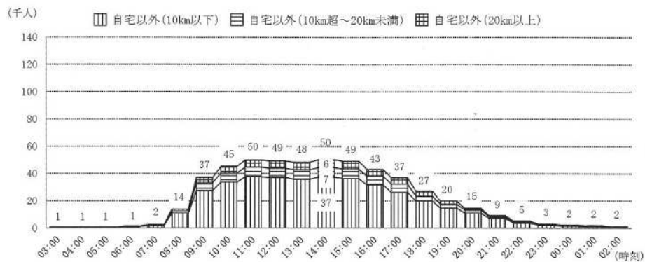
図 主要ゾーンの時刻別自宅までの距離帯別滞留人口(平日)
