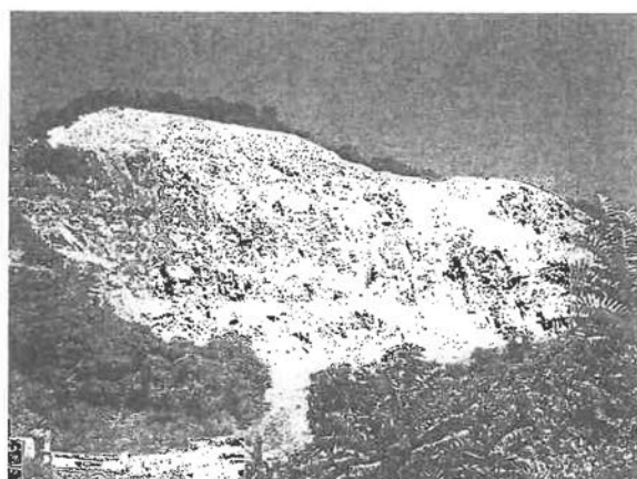
写真1 岡山市東区瀬戸町の採石場 急流小河川の中腹部にあり、下流に人家や県道がある。最上部に3段の段切りをしているが現在急立した崖の下から掘り進んでいる。
