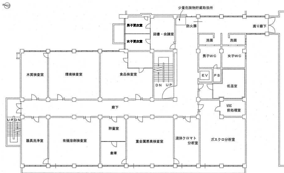
2 階平面図
