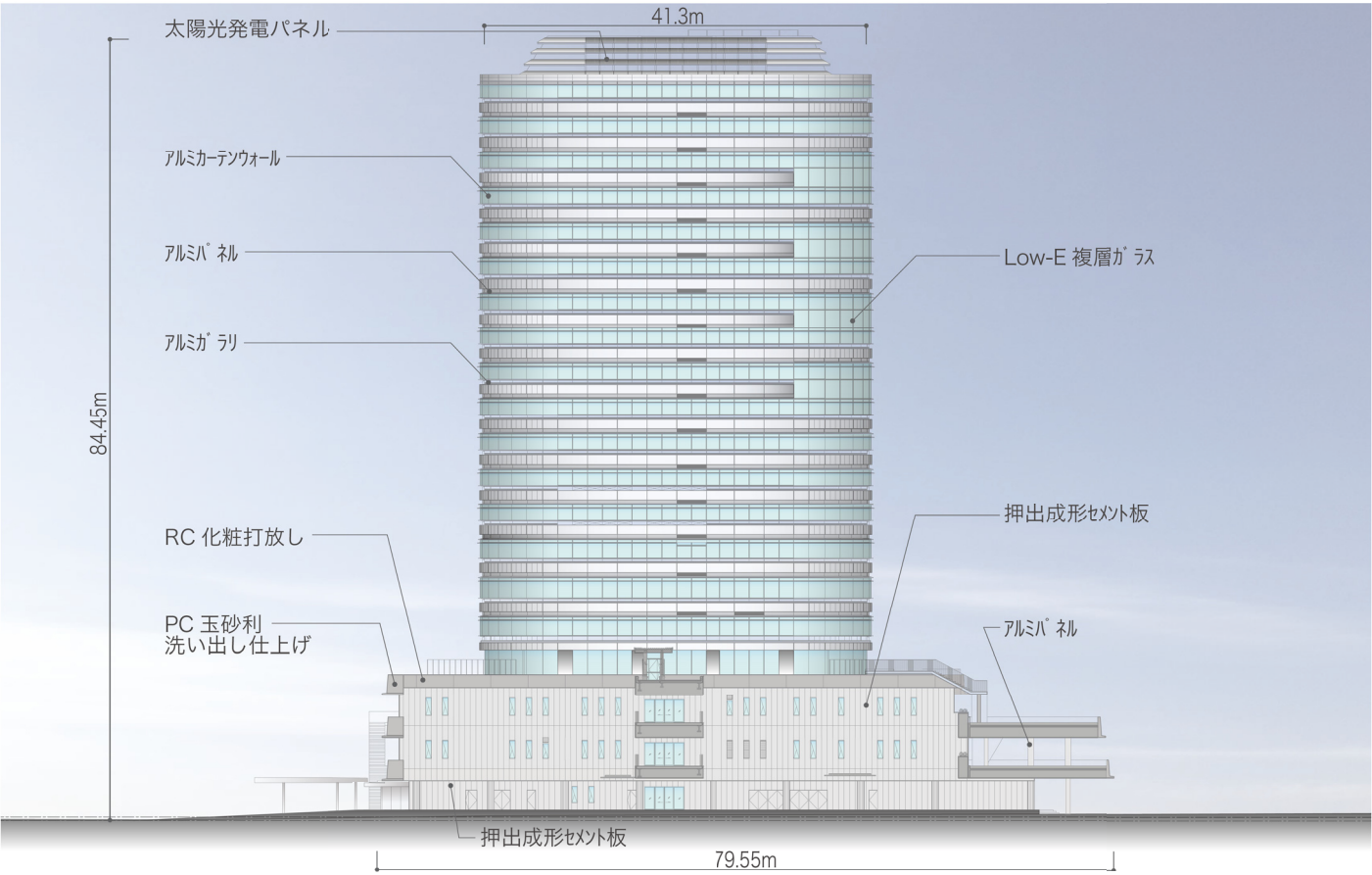
■ 西側立面図
