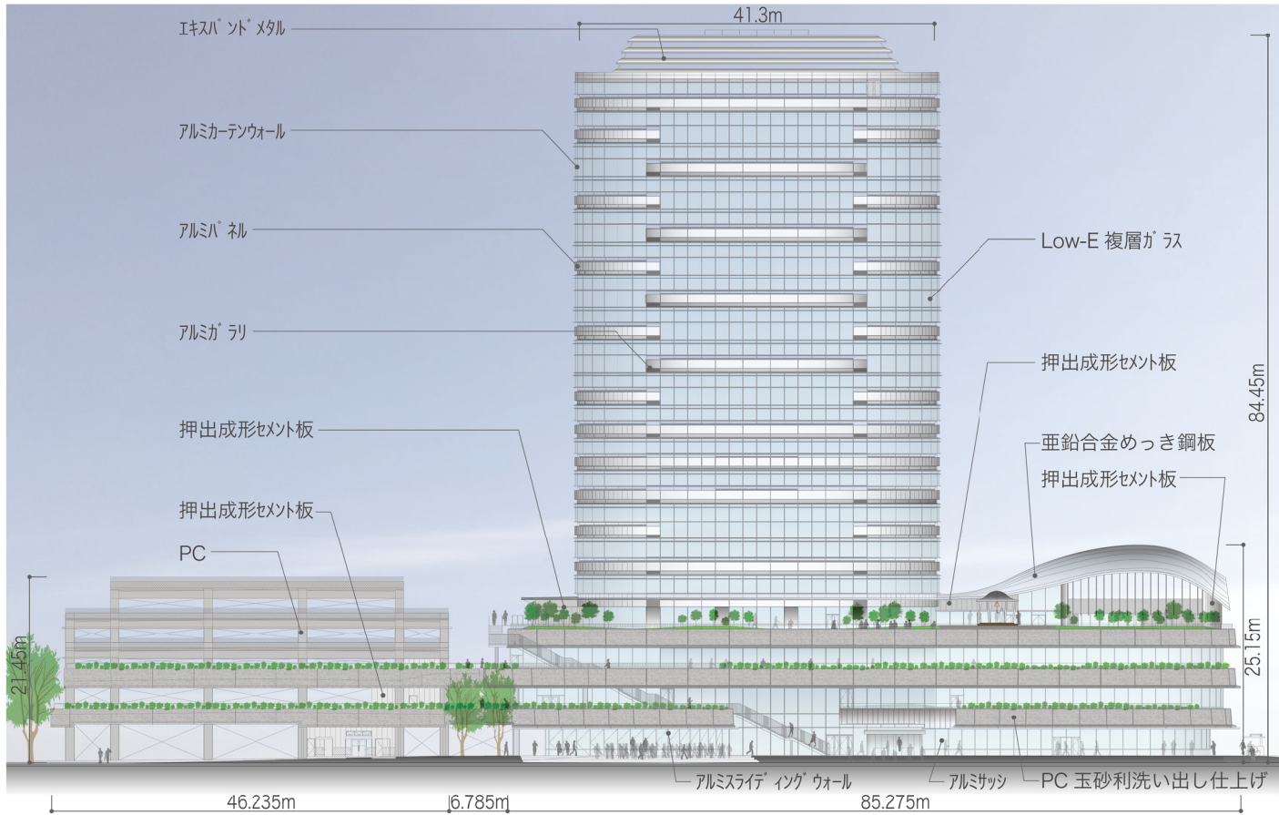
■ 北側立面図
