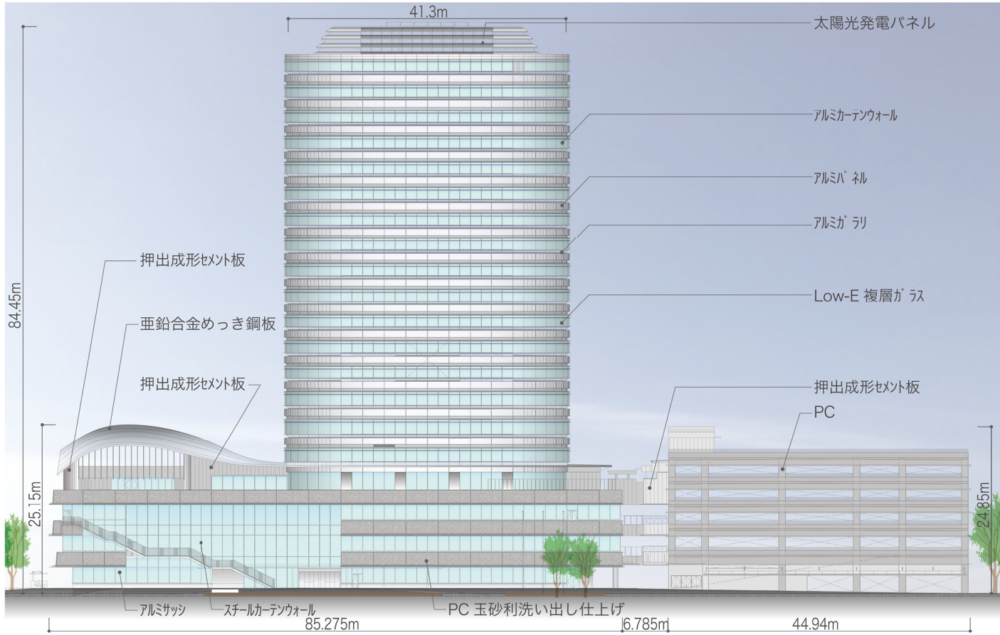
■ 北側立面図
