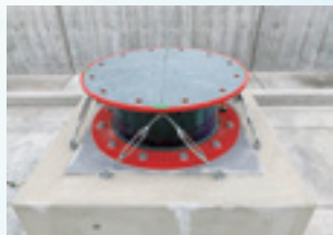
▲写真①(積層ゴム支承)
