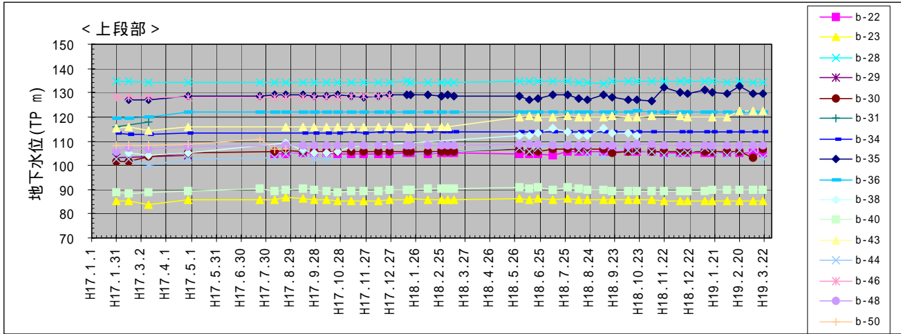
図 3.4.8 地下水位の経時変化
