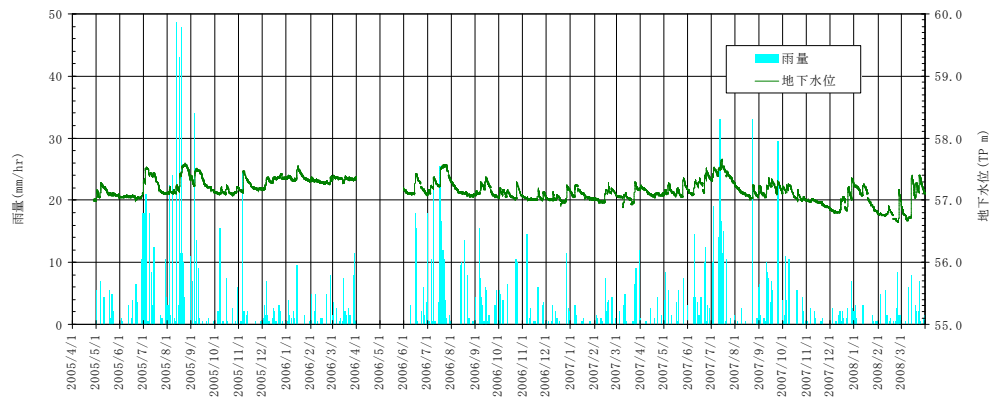
雨量と水位変動(BW-02)
