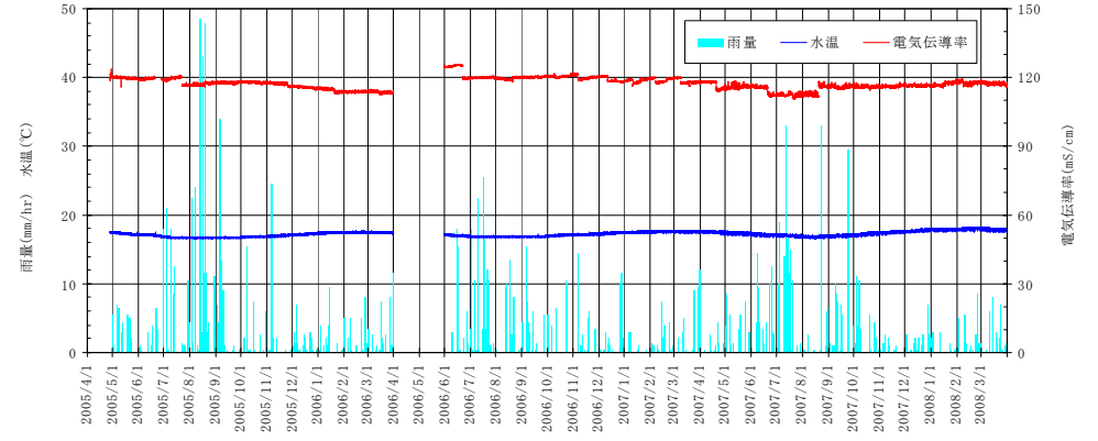
降雨量と電気伝導率変動(BW-01)
