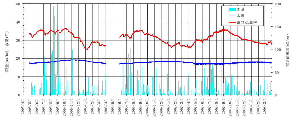
降雨量と電気伝導率(BW-02)
