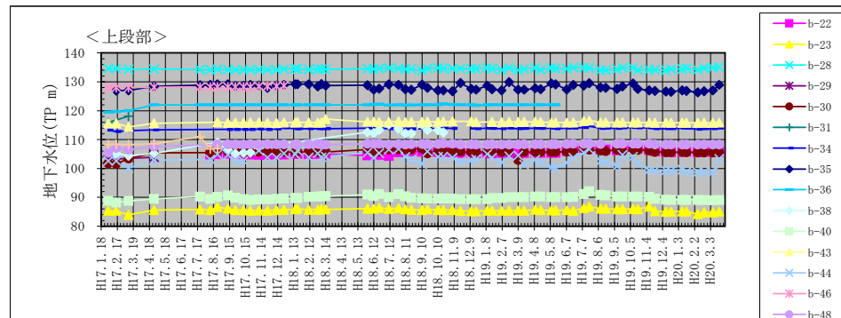
地下水位の経時変化
