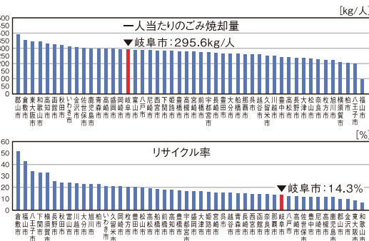
図92 中核市の一人当たりのごみ焼却量及びリサイクル率(2015年度) 出典:一般廃棄物処理実態調査(環境省)
