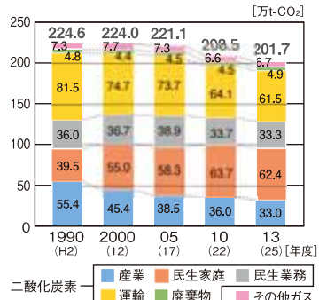
図93 市の温室効果ガス排出量の推移
