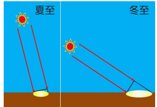
図1：太陽の光のあたり方のちがいを
