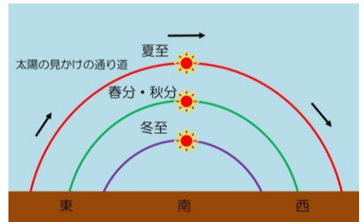
図2：地上から見た太陽の通り道
