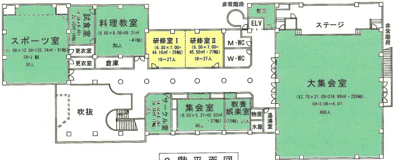
2階平面図
