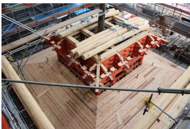
初重の野地板を貼り終わりました。7月からは三重の柱、梁の組立てに取り掛かります。
