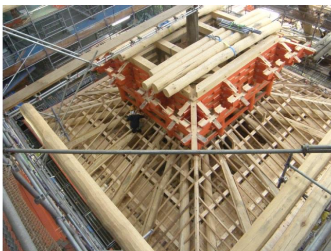
桔木と補強金物の設置が完了し屋根の垂木を設置します。
