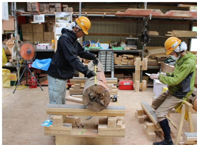
三重の柱を修復しています。(既設部材)
