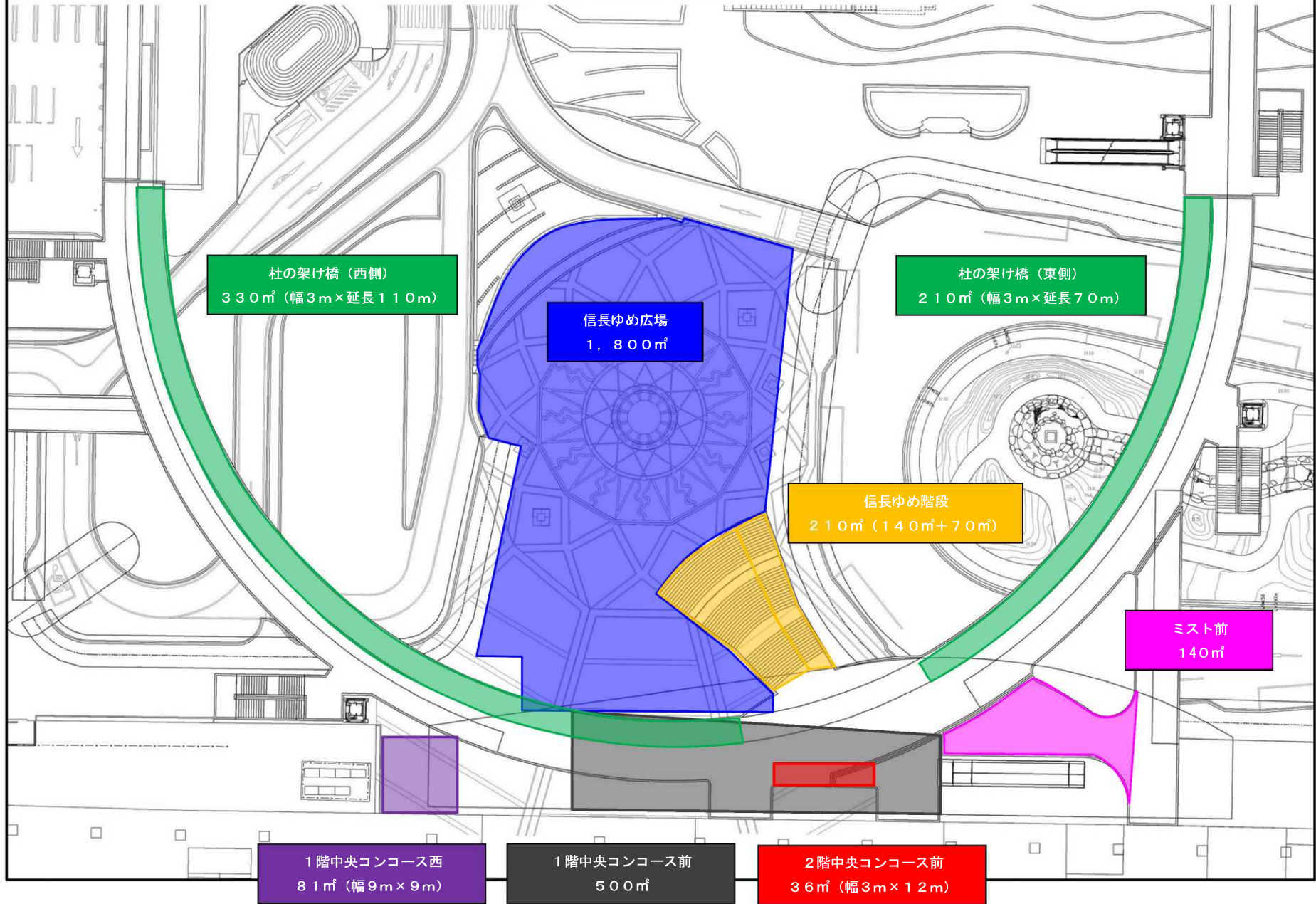
岐阜駅北口駅前広場平面図
