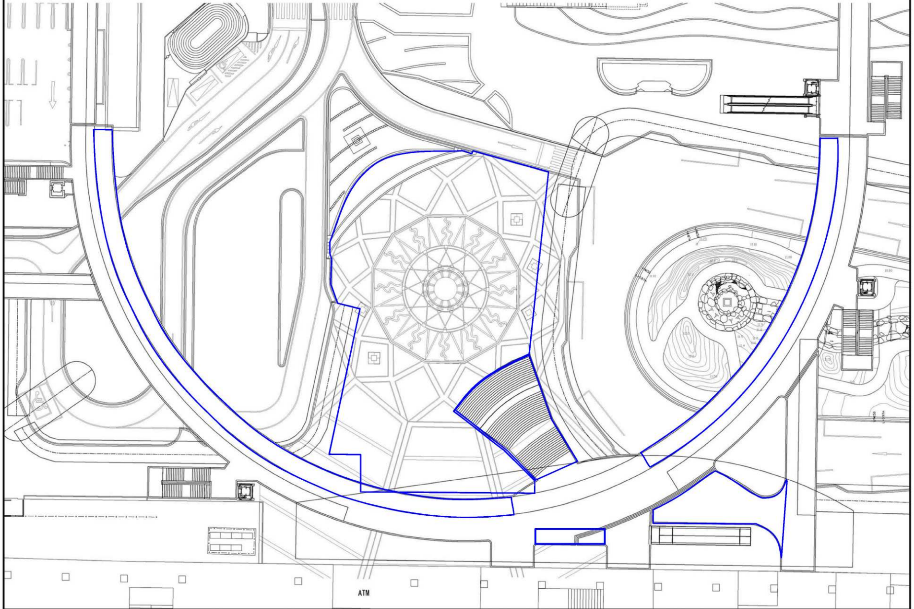
岐阜駅北口駅前広場平面図
