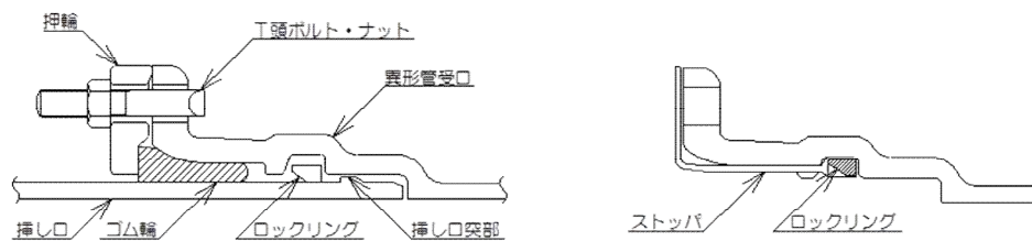
図4-11 GX形異形管の接合
