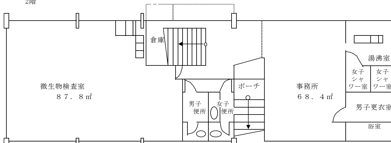
1階
