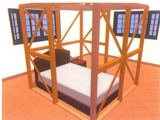
耐震ベッド(一例)
