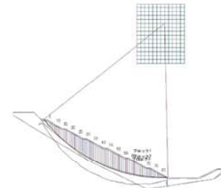
B-13 レベル1地震動(Kh=0.08)
