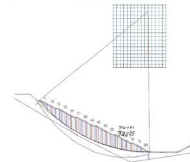
B-13 レベル2地震動(Kh=0.16)
