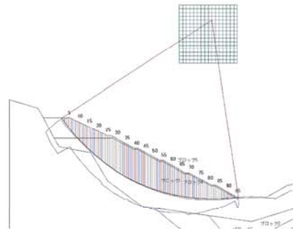
B-10 レベル1地震動(Kh=0.08)
