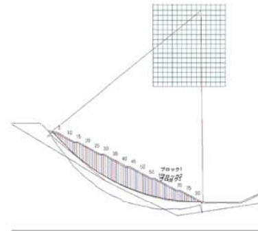
B-13 レベル2地震動(Kh=0.16)
