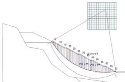
B-10 レベル2地震動(Kh=0.16)
