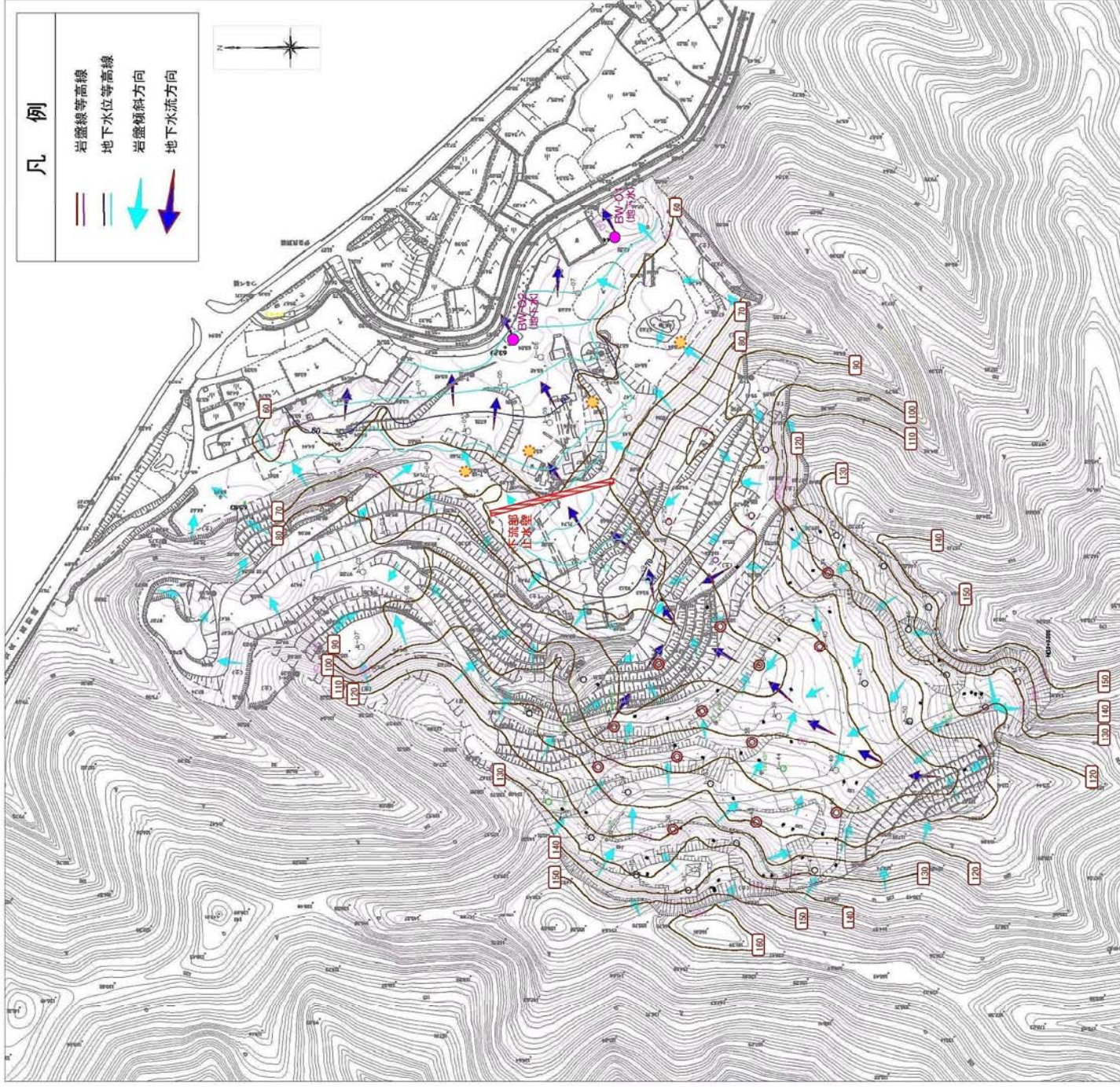
岩盤等高線と地下水位
